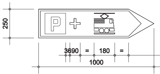
Abb. 13 Wegweiser «Parkplatz mit Anschluss an öffentliches Verkehrsmittel» (Beispiel) (Sig. 4.46.1)
