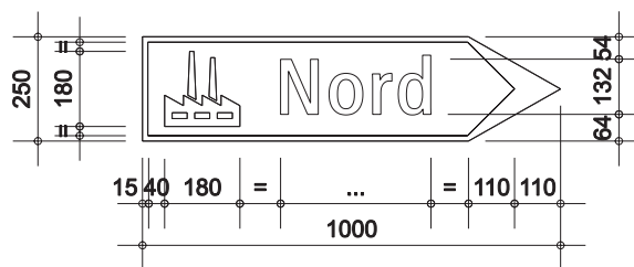
Abb. 17b Sammelwegweiser für Industrie- und Gewerbebezonen Beispiel mit Symbol «Industrie- und Gewerbegebiet» und Gebietsname
