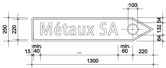
Fig. 16 Indicateur de direction «Entreprise» (sig. 4.49)
