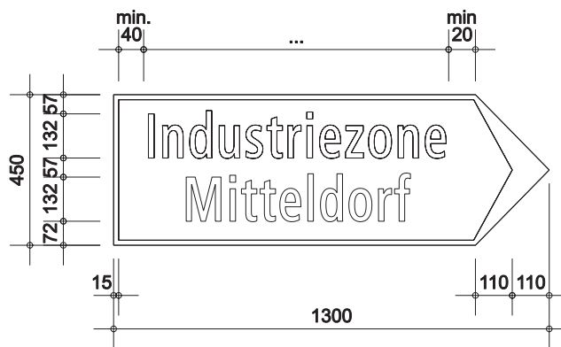
Abb. 17a Sammelwegweiser für Industrie- und Gewerbebezonen Beispiel mit Sammelbegriff und Gebietsname
