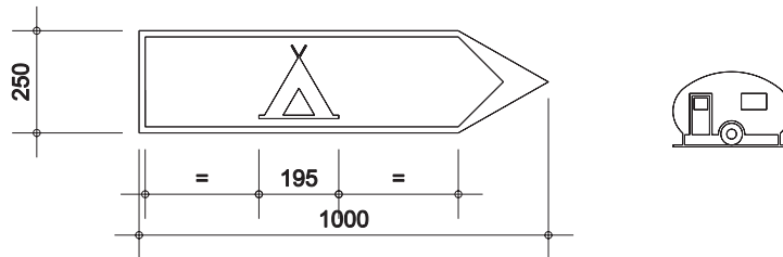
Fig. 14 Indicateur de direction «Place de camping» (sig. 4.47) Indicateur de direction «Terrain pour caravanes» (sig. 4.48)
