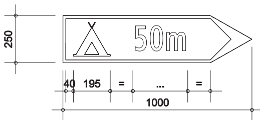
Abb. 15 Wegweiser «Zeltplatz» mit Distanzangabe (Sig. 4.47)
